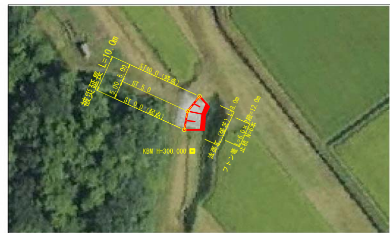
平面図 S=1:500
