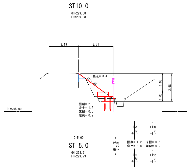
構造図
