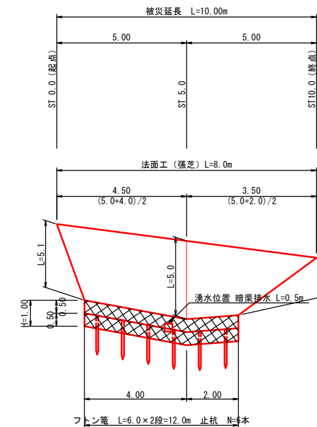
展開図 S=1:100
