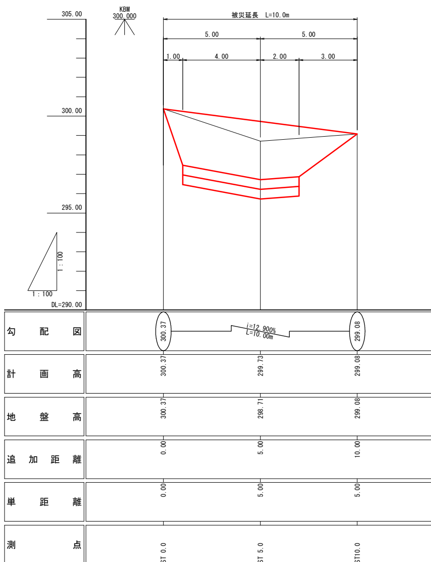
縦断面 V=1:100 H=1:100
