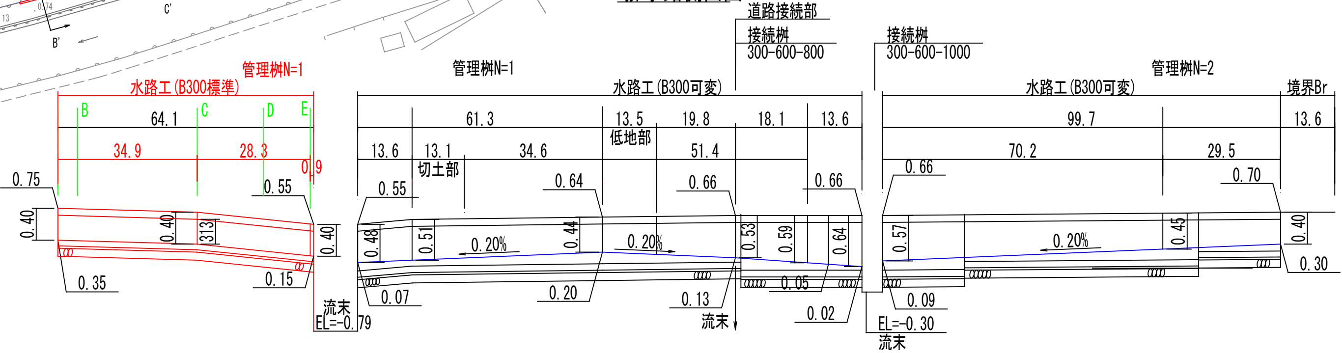
排水路側面図
