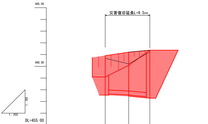
縦断図
