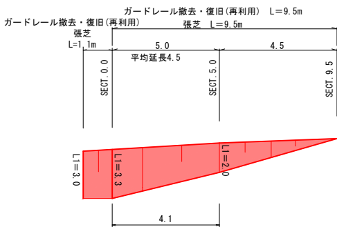
展開図
