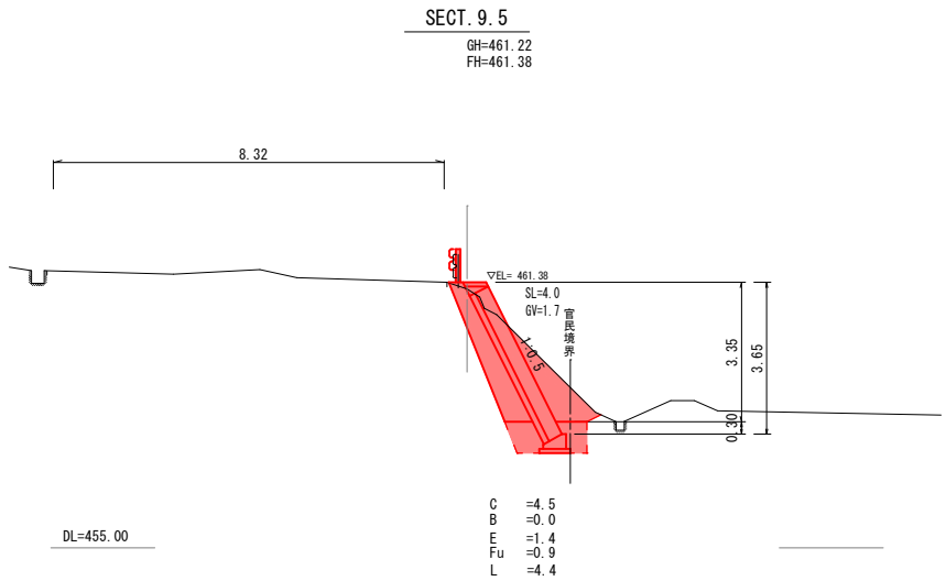
横断図
